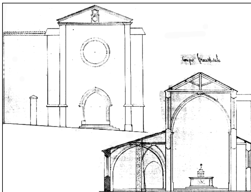
Plan, coupe et élévation de l'église saint-Pierre de Montbrison du 5 mars 1836
