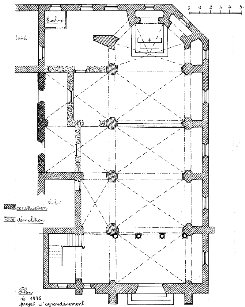
Plan de l'église Saint-Pierre de Montbrison
